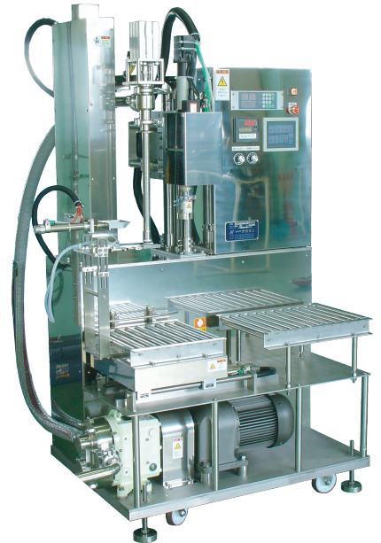
半自動バックインボックス充填機 (アンキャッパー／キャッパー付き)
