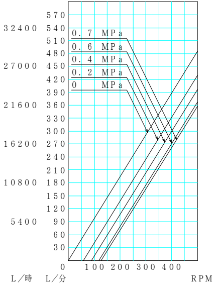
液名: 水 機種: JMU125 液質: 1mPa·s 配管径: 2 1/2"
