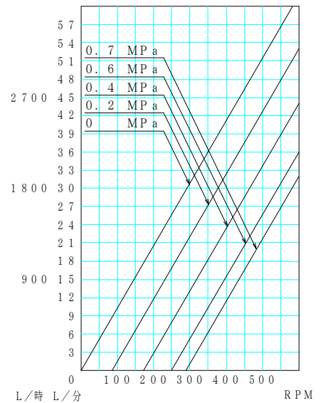
液名: CMC水溶液 機種: JMU55 液質: 500mPa·s 配管径: 2"
