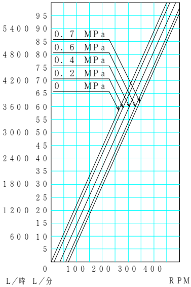
液名: CMC水溶液 機種: JMU125 液質: 500mPa·s 配管径: 2 1/2"
