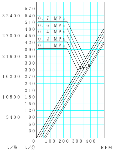
液名: CMC水溶液 機種: JMU125 液質: 500mPa·s 配管径: 2 1/2"
