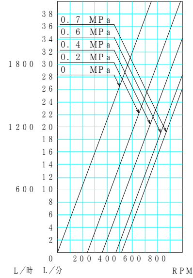
液名: 水 機種: JMU40 液質: 1mPa·s 配管径: 2"
