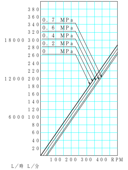
液名: CMC水溶液 機種: JMU200 液質: 500mPa·s 配管径: 4"
