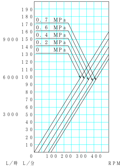
液名: CMC水溶液 機種: JMU160 液質: 500mPa·s 配管径: 4"
