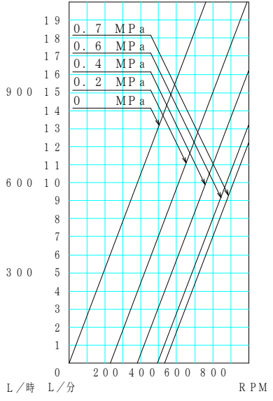
液名: 水 機種: JMU25 液質: 1mPa·s 配管径: 1 1/2"
