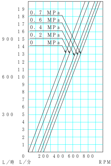
液名: CMC水溶液 機種: JMU25 液質: 500mPa·s 配管径: 1 1/2"
