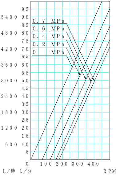
液名: 水 機種: JMU125 液質: 1mPa·s 配管径: 2 1/2"
