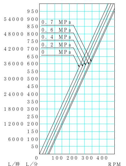
液名: CMC水溶液 機種: JMU200 液質: 500mPa·s 配管径: 4"
