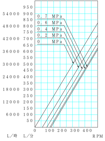
液名: 水 機種: JMU160 液質: 1mPa·s 配管径: 4"
