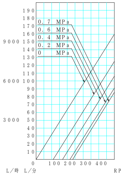
液名: 水 機種: JMU160 液質: 1mPa·s 配管径: 4"
