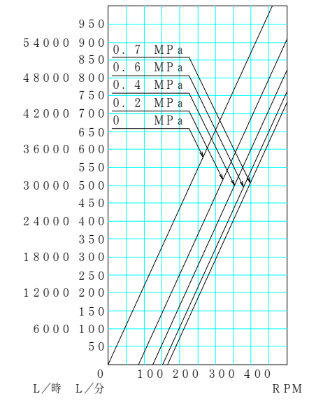
液名: 水 機種: JMU200 液質: 1mPa·s 配管径: 4"
