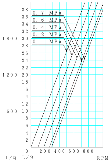
液名: CMC水溶液 機種: JMU40 液質: 500mPa·s 配管径: 2"
